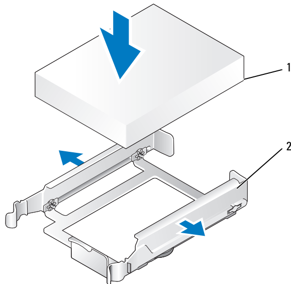
1 Festplatte 2 Festplattenlaufwerkhalterung
